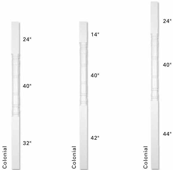
W-3048-4" W-3058-5" W-3068-6"
